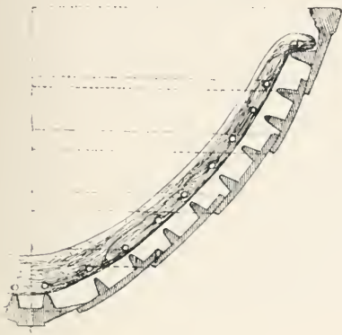
329a. Durchschnitt des Schiffes Fig. 329.
